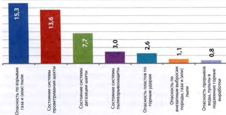
Рис. 2. Затраты на выполнение мероприятий по повышению безопасности на шахтах на период до 2020 года, млрд руб.
